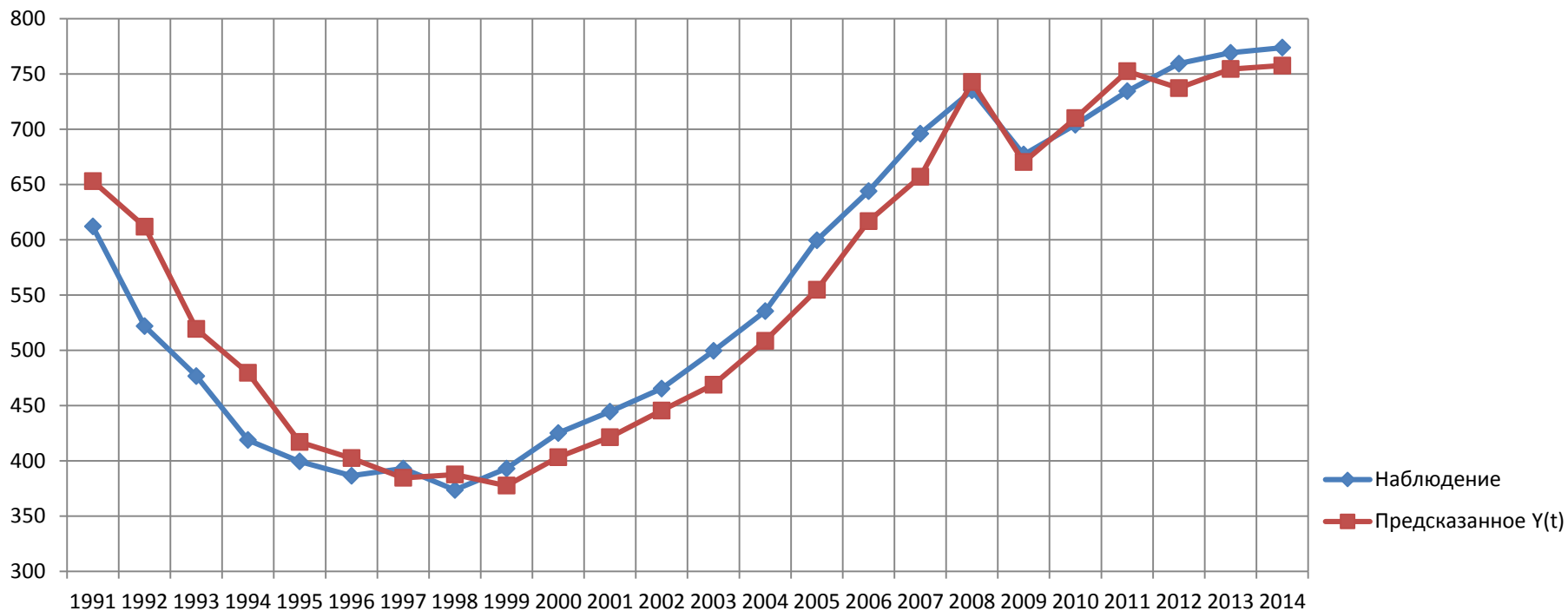
Рис. 5 Российский ВВП как регрессия от прошлогоднего ВВП и годовой разности цен на экспортируемую нефть Y(t) = 1,000457Y(t-1) + 0,000344 [p(t)-p(t-1)] Y(t-1) R=0,998428; R^2= 0,996858; R^2_{norm}= 0,95126 t\text{-статистика: } 80,35; 3,03.
