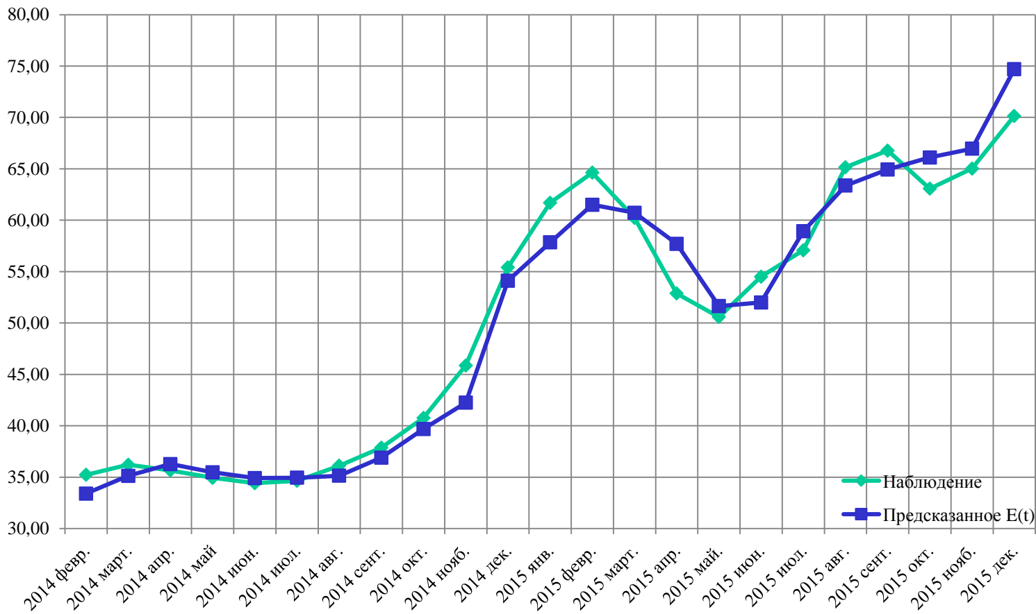
Рис.4. Обменный курс руб./дол. как разностная регрессия от цены нефти Брент P и учетной ставки Центробанка S .
