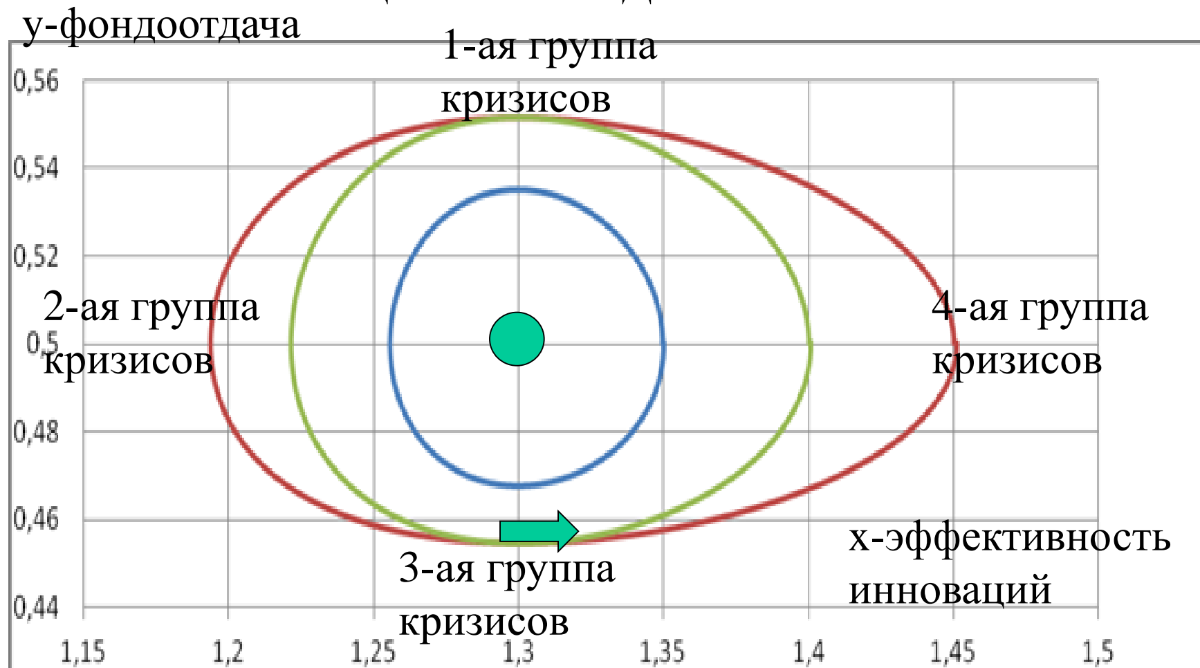
Рис.2 . Равновесное состояние x=1,3 , y=0,5 ; орбиты с периодами 50,1 г., 54,9 г., 60,6 г.. Движение против часовой стрелки.
